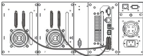
Рисунок 3. Кабельные соединения SCSI для двух устройств
